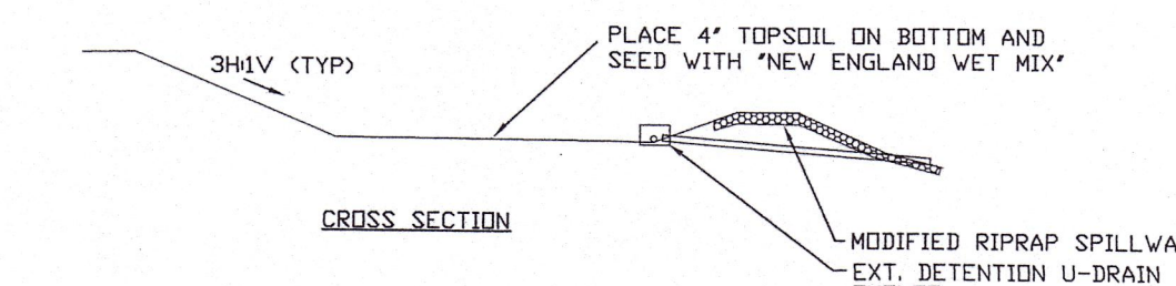
WATER QUALITY BASIN (N.T.S.)
