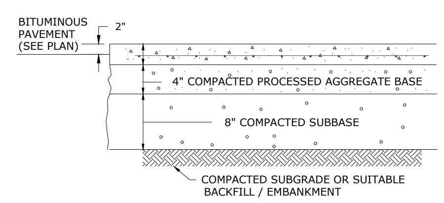
CONCRETE PAD SCALE: NONE
